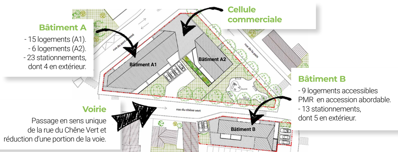
Plan de masse global sur le périmètre de la Croix Hubin
